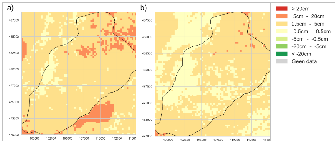
Figuur 5.25 Het effect op de grondwaterstand (GLG) van de toepassing van brakwaterwinning (50% van de kwel) met in a) zonder infiltratie van het concentraat en in b) met concentraatinfiltratie (25% van de kwel) ten opzichte van de referentiesituatie (zonder afvangen van brakke kwel) in de Haarlemmermeerpolder.
