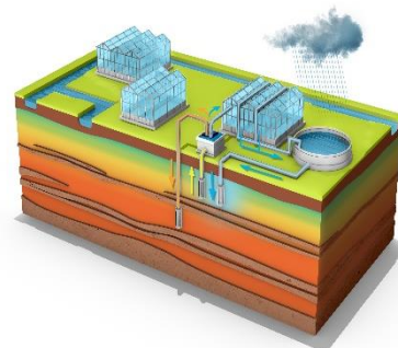
Figuur 2.2 Voorbeeld van ondergrondse opslag van zoetwater
