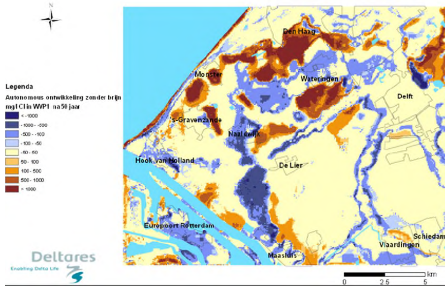
FIGUUR 2-4: VERANDERING AUTONOME CHLORIDE CONCENTRATIES (EERSTE WATERVOERENDE PAKKET) IN HET WESTLAND IN 50 JAAR (SINDS 2010) (FANECA SÁNCHEZ ET AL., 2012).
