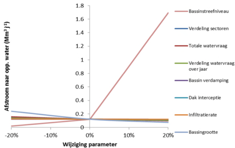
FIGUUR 5-8. GEVOELIGHEIDSANALYSE VAN DE HOEEVEELHEID WATER DIE NAAR HET OPPERVLAKTEWATER AFSTROOMT IN MILJOEN M^3 J^{-1} , UITGAANDE VAN EEN GEMIDDELTE WATERVRAAG VAN 682 MM/J.
