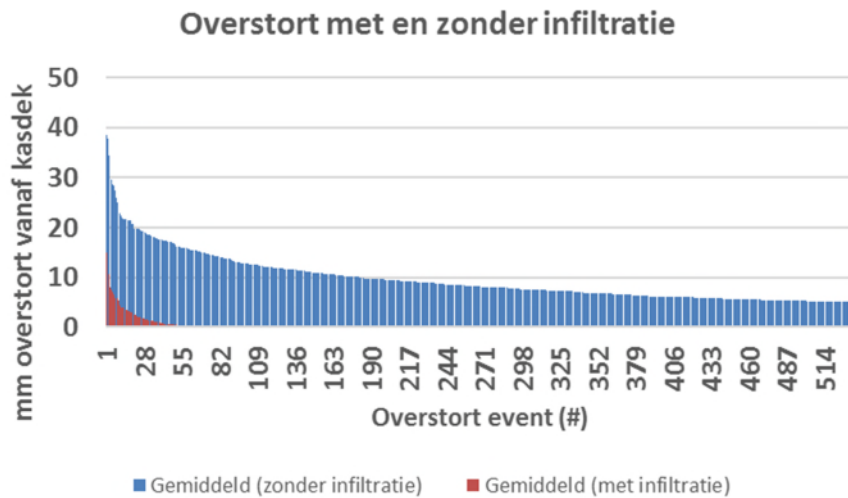
FIGUUR 5-11. OVERSTORT (GEMIDDELD) PER EVENT MET EN ZONDER INFILTRATIE CF. AANGENOMEN REGIME. WATERVRAAG: 682 MM/J
