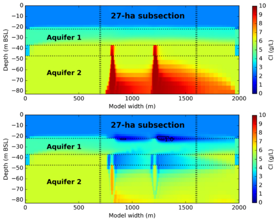
FIGUUR 3-3. DOORSNEDEN VAN DE GEMODELLEERDE GEMIDDELDE CHLORIDECONCENTRATIES IN HET GRONDWATER NA 30 JAAR BRAKWATERWINNING (RO, BOVEN) EN 30 JAAR ONDERGRONDSE WATERBERGING IN COMBINATIE MET BRAKWATERWINNING (ASR+RO, ONDER). OP BASIS VAN DE LOCATIE PROMINENT GROENEWEG (ROS AND ZUURBIER, 2017).
