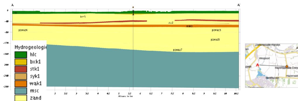
FIGUUR 4-10. DOORSNEDE VAN DE ONDERGROND IN DE POLDER DE NOORDPLAS (REGIS).
