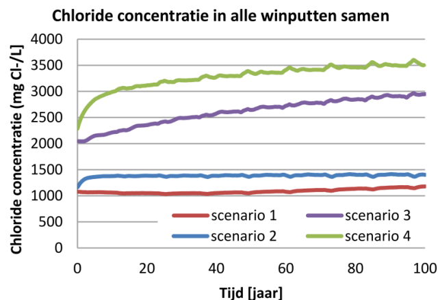
FIGUUR 4-27. ZOUTCONCENTRATIE OVER DE KOMENDE 100 JAAR IN ALLE WINPUTTEN VOOR SCENARIO 1, 2, 3 EN 4 OP DEZELFDE RUIMTELIJKE LOCATIES (MET ALS VERSCHIL DAT DE WINPUTTEN VAN SCENARIO 3 EN 4 DIEPER LIGGEN).
