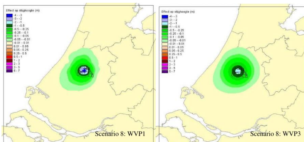
FIGUUR 4-6. EFFECTEN VAN WINNING (EN AFVOER VAN BRAKWATER UIT HET GEBIED) VAN 25 MILJOEN \text{M}^3/\text{JAAR} OP DE STIJGHOOGTEN IN HET EERSTE EN DERDE WATERVOERENDE PAKKET (DE LOUW ET AL., 2007).
