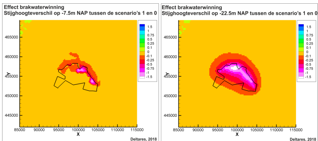
FIGUUR 4-18. VERANDERINGEN IN STIJGHOOGTE IN DE OMGEVING VAN DE POLDER DE NOORDPLAS ALS GEVOLG VAN DE BRAKWATERWINNINGEN VAN SCENARIO 1. LINKS: VERSCHIL IN STIJGHOOGTE TUSSEN HET REFERENTIE SCENARIO 0 EN SCENARIO 1 IN HET EERSTE WATERVOEREND PAKKET (-7.5m NAP); RECHTS: IDEM IN HET TWEEDE WATERVOEREND PAKKET (-22.5m NAP).
