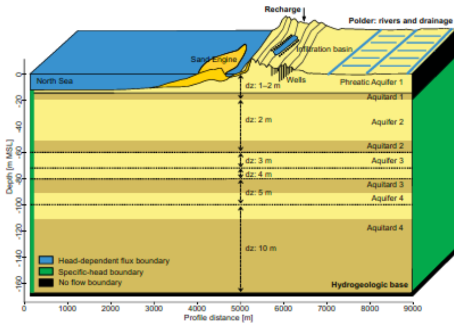
FIGUUR 3-3. SCHEMATISATIE VAN HET GRONDWATERMODEL UIT: (HUIZER ET AL., 2016). NB: LET OP VERSCHIL IN SCHAALEN HORIZONTAAL (9 KM) / VERTICAAL (160 M).
