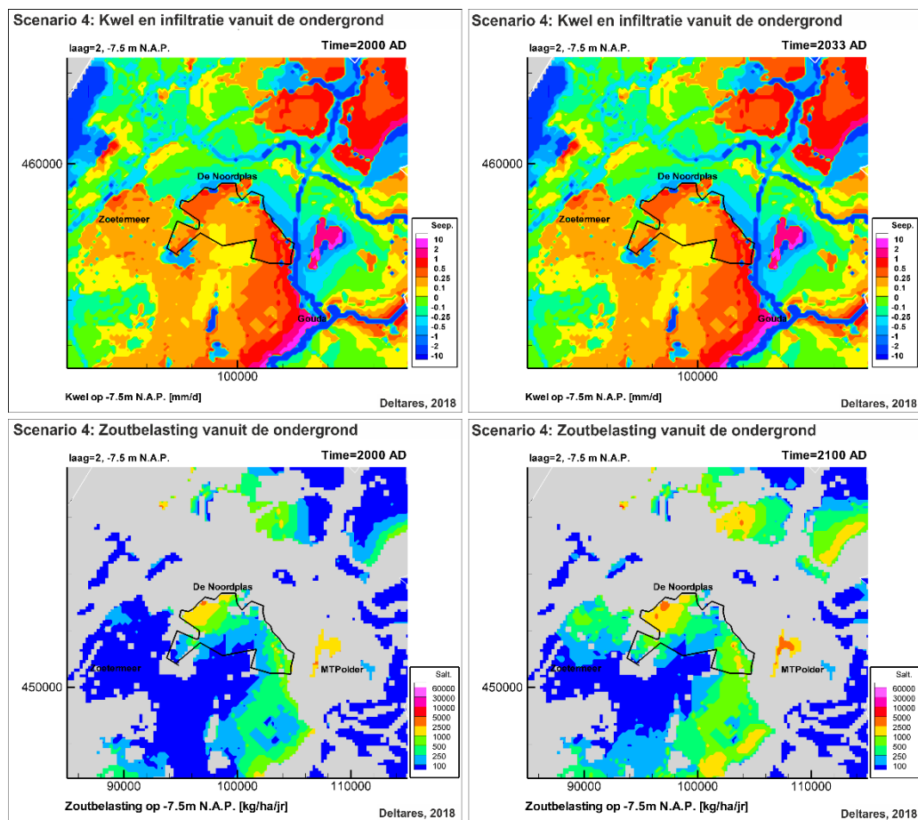
FIGUUR 4-22. EFFECT VAN BRAKWATERWINNING, SCENARIO 4: VERANDERING KWEL/INFILTRATIE (BOVEN) EN ZOUTVRACHT (ONDER) IN DE HUIDIGE SITUATIE (LINKS) EN OVER DE KOMENDE 100 JAAR (RECHTS).
