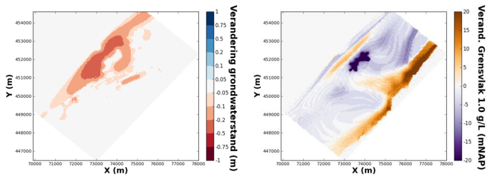
FIGUUR 3-14: LINKS: VERANDERING GRONDWATERSTAND TEN OPZICHTE VAN REFERENTIE SCENARIO, 2050. RECHTS: VERANDERING POSTIE ZOET-ZOUT GRENSVLAK (1.0 G/L) TEN OPZICHTE VAN REFERENTIE SCENARIO, 2050.
