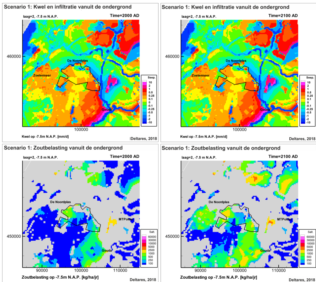
FIGUUR 4-17. EFFECT VAN BRAKWATERWINNING, SCENARIO 1: VERANDERING KWEL/INFILTRATIE (BOVEN) EN ZOUTVRACHT (ONDER) IN DE HUIDIGE SITUATIE (LINKS) EN OVER DE KOMENDE 100 JAAR (RECHTS).
