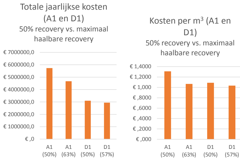
FIGUUR 6-5. TOTALE JAARLIJKSE KOSTEN EN KOSTEN PER M 3 VERGELEKEN VOOR SCENARIO A1 EN D1 BIJ VERSCHILLENDE RO RECOVERY EFFICIENCIES. RENTE: 3%
