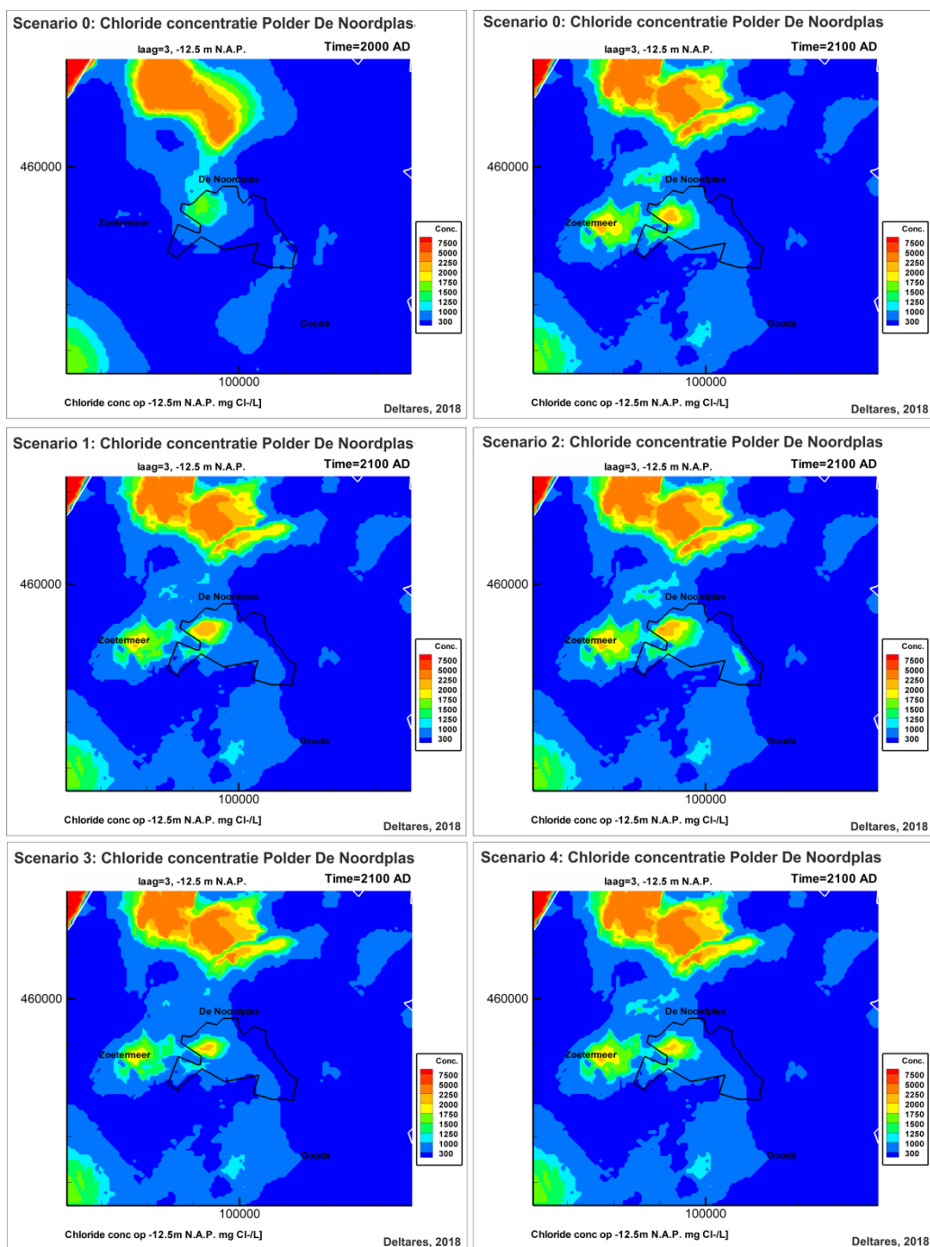
FIGUUR 4-24. EFFECT VAN VERSCHILLENDE SCENARIO'S OP DE ZOET-ZOUT VERDELING IN DE ONDERGROND, NAAST ONTWIKKELING VAN DE REFERENTIE SITUATIE (HUIDIG EN OVER 100 JAAR): BOVENAANZICHT CHLORIDE CONCENTRATIE OP -12.5M NAP.
