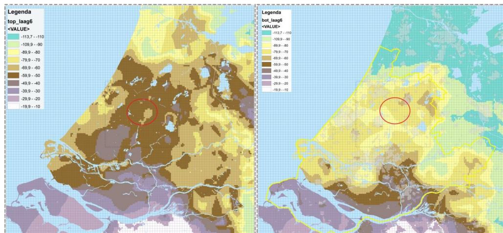
FIGUUR 4-14. DE DIEPTELIGGING VAN DE BOVEN- (LINKS) EN ONDERKANT (RECHTS) VAN HET TWEDE WATERVOERENDE PAKKET, OMCIRKELD IS DE LOCATIE VAN POLDER DE NOORDPLAS.
