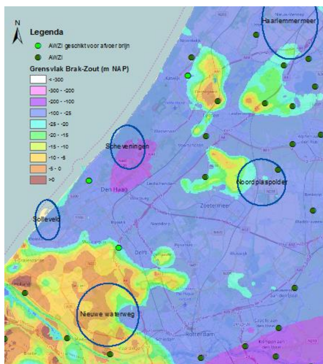
FIGUUR 2-1. DIEPTÉ VAN HET BRAK-ZOUT GRENSVLAK ( 1000 \text{ mg L}^{-1} \text{ Cl}^{-1} ) IN METERS TEN OPZICHT VAN NAP (OUDE ESSINK ET AL. 2010).
