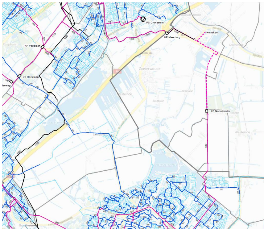
FIGUUR 5-4. LIGGING BELANGRIJKSTE INFRASTRUCTUUR RUWATER (ZWART) EN REINWATER (PAARS EN BLAUW) DUNEA
