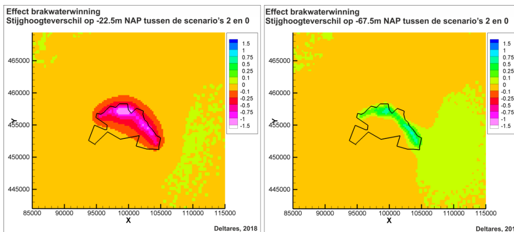
FIGUUR 4-20. VERANDERINGEN IN STIJGHOOGTE IN DE OMGEVING VAN DE POLDER DE NOORDPLAS ALS GEVOLG VAN DE BRAKWATERWINNINGEN VAN SCENARIO 2. LINKS: VERSCHIL IN STIJGHOOGTE TUSSEN HET REFERENTIE SCENARIO 0 EN SCENARIO 2 IN HET EERSTE WATERVOEREND PAKKET (-22.5M NAP); RECHTS: IDEM IN HET TWEEDE WATERVOEREND PAKKET (-67.5M NAP).
