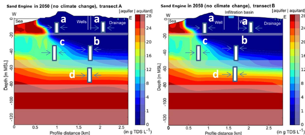
FIGUUR 3-6: POTENTIËLE WINLOCATIES BRAKWATER IN DE ZOETWATERLENS BIJ SOLLEVELD IN EEN DWARDSDOORSNEDE.
