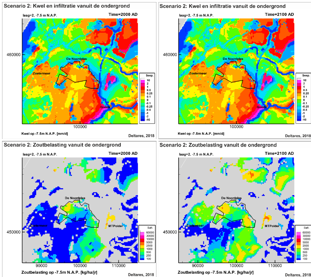
FIGUUR 4-19. EFFECT VAN BRAKWATERWINNING, SCENARIO 2: VERANDERING KWEL/INFILTRATIE (BOVEN) EN ZOUTVRACHT (ONDER) IN DE HUIDIGE SITUATIE (LINKS) EN OVER DE KOMENDE 100 JAAR (RECHTS).
