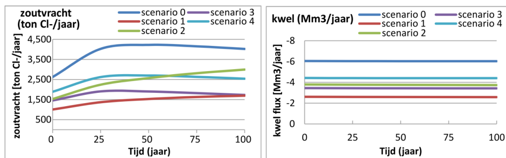
FIGUUR 4-26. ONTWIKKELING IN ZOUTVRACHT EN KWEL PER SCENARIO GEDURENDE DE KOMENDE 100 JAAR.
