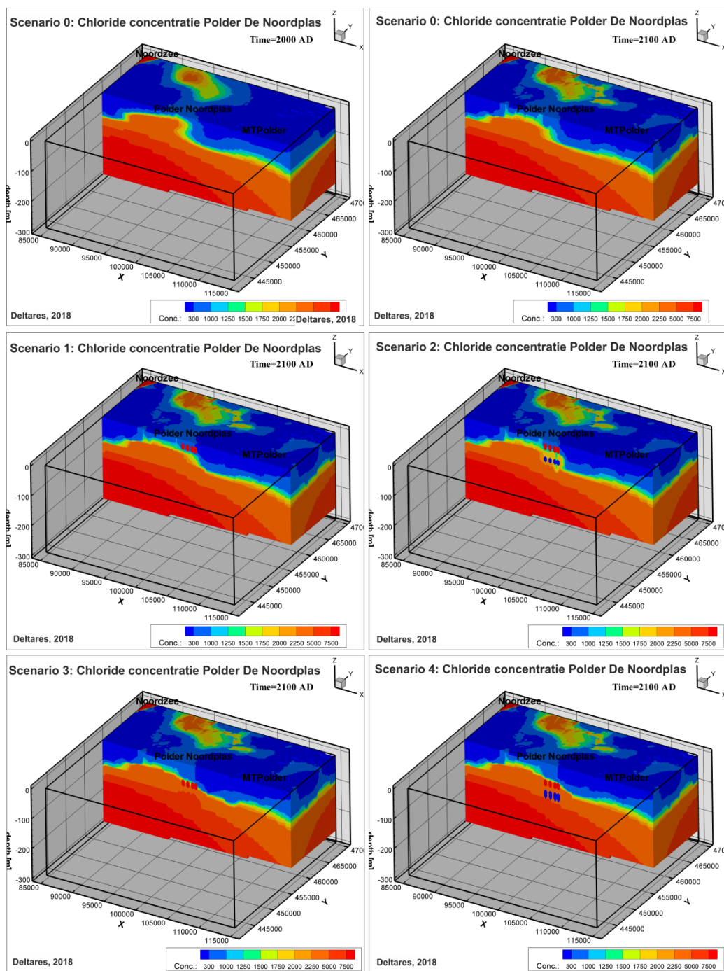
FIGUUR 4-23. EFFECT VAN VERSCHILLENDE SCENARIO'S OP DE ZOET-ZOUT VERDELING IN DE ONDERGROND, NAAST DE ONTWIKKELING VAN DE REFERENTIE SITUATIE (EERSTE RIJ: HUIDIG LINKS EN OVER 100 JAAR RECHTS): LOCATIES WINPUTTEN TE HERKENNEN AAN RODE (ONTTREKKING) EN BLAUWE (INFILTRATIE) PUNTEN.
