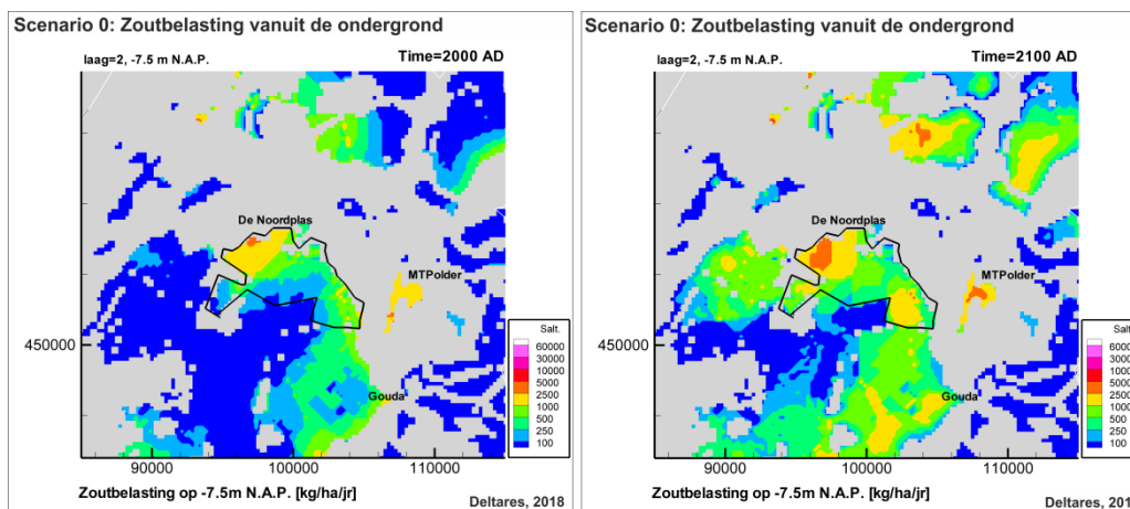
FIGUUR 4-16. ZOUTVRACHT VANUIT DE ONDERGROND IN DE REGIO VAN DE POLDER DE NOORDPLAS: LINKS DE HUIDIGE ZOUTVRACHT IN HET SCENARIO 0 (REFERENTIESITUATIE), EN RECHTS: DE TOEKOMSTIGE ZOUTVRACHT IN HET SCENARIO 0 (REFERENTIESITUATIE) OVER 100 JAAR.
