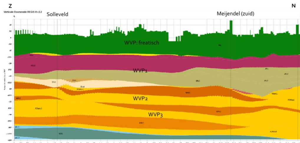
FIGUUR 3-18. DOORSNEDEN GEOLOGISCH PROFIEL (LITHOLOGISCHE KARAKTERISATIE) ZUID-NOORD REGIS II 2.2.
