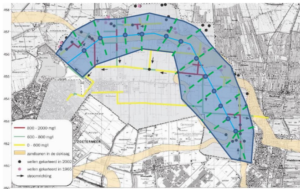
FIGUUR 4-11. POTENTIËLE ZONE VOOR BRAK GRONDWATER ONTTREKKING IN DE POLDER DE NOORDPLAS (MET PUTTENVELD BESTAANDE UIT HORIZONTALE PUTTEN TER ILLUSTRATIE).
