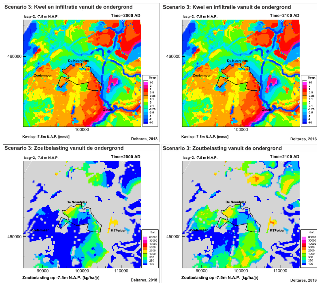
FIGUUR 4-21. EFFECT VAN BRAKWATERWINNING, SCENARIO 3: VERANDERING KWEL/INFILTRATIE (BOVEN) EN ZOUTVRACHT (ONDER) IN DE HUIDIGE SITUATIE (LINKS) EN OVER DE KOMENDE 100 JAAR (RECHTS).
