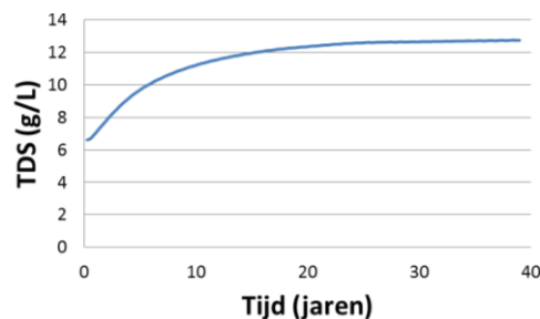
FIGUUR 3-13. VERLOOP VAN DE CHLORIDE CONCENTRATIE VAN HET ONTTROKKEN WATER IN ADDITIONELE WINNINGEN IN SCENARIO 3.
