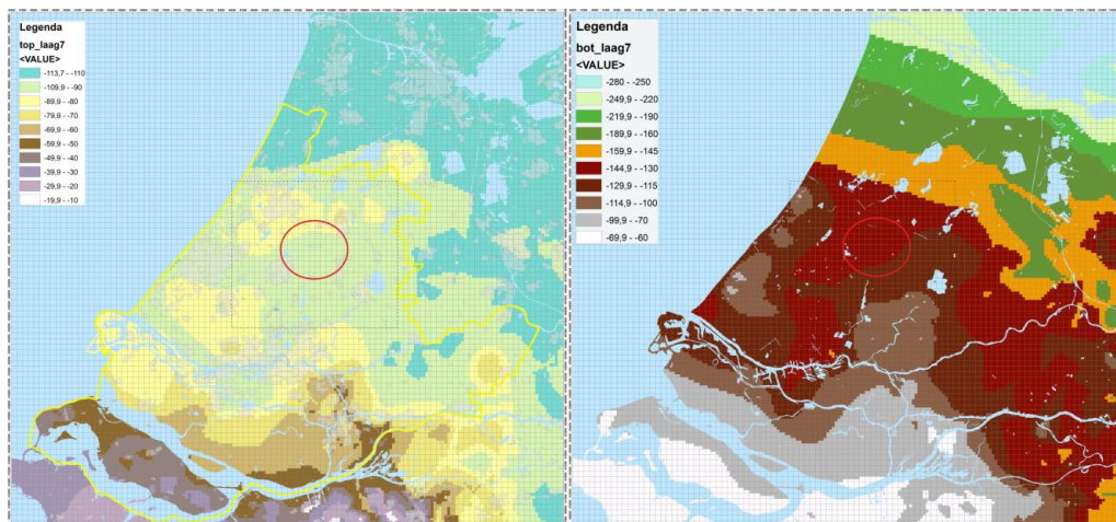
FIGUUR 4-15. DE DIEPTELIGGING VAN DE BOVEN- (LINKS) EN ONDERKANT (RECHTS) VAN HET DERDE WATERVOERENDE PAKKET, OMCIRKELD IS DE LOCATIE VAN DE POLDER DE NOORDPLAS.
