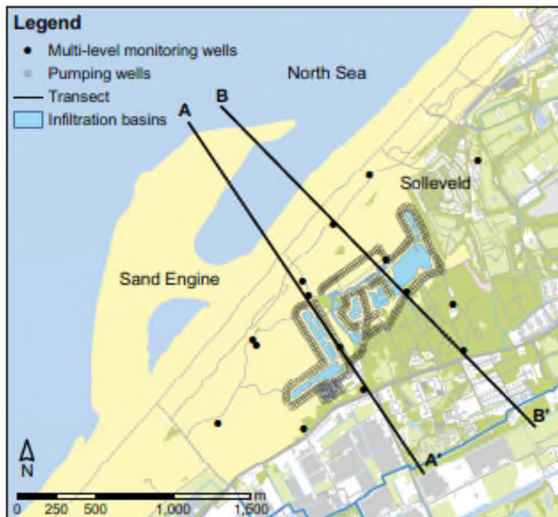
FIGUUR 3-1. DUINGEBIED SOLLEVELD NABIJ DE ZANDMOTOR, MET DE INFILTRATIEVIJVERS, WIN- EN MONITORINGSPUTTEN (UIT: HUIZER ET AL. (2016)).
