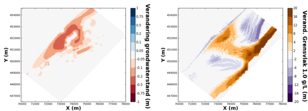
FIGUUR 3-10: LINKS: VERANDERING GRONDWATERSTAND TEN OPZICHT VAN REFERENTIE, 2050. RECHTS: VERANDERING POSITIE ZOET-ZOUT GRENSVLAK (1.0 g/L) TEN OPZICHT VAN REFERENTIE, 2050.
