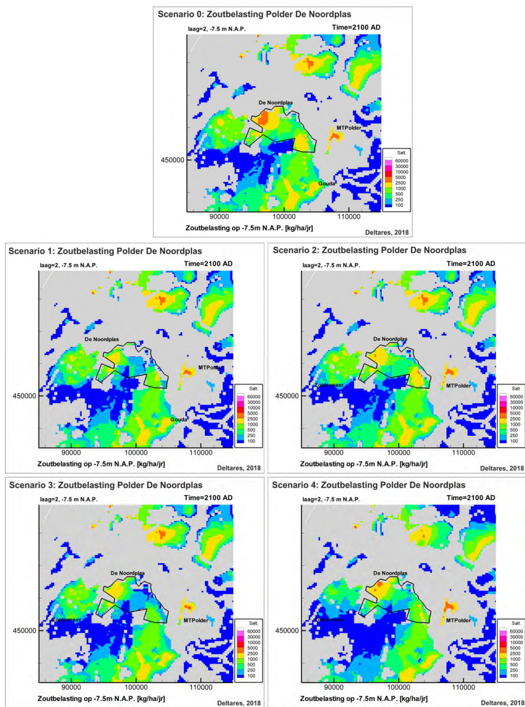
FIGUUR 4-25. EFFECT VAN DE BRAKWATERWINNING OP DE ZOUTVRACHT (BOVEN: SCENARIO 1 (LINKS) EN SCENARIO 2 (RECHTS) EN ONDER: SCENARIO 3 (LINKS) EN SCENARIO 4 (RECHTS)).
