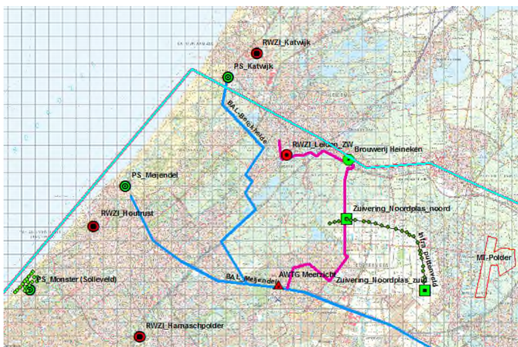
FIGUUR 5-3. LIGGING POMPSTATIONS, RWZI'S, RELEVANT LEIDINGWERK EN DE MOGELIJKE INRICHTING VAN DE WINNING NOORDPLAS. NB: BAL IS DUBBEL UITGEVOERD TOT SPLITSING MEIJENDEL/BERCKHEIDE
