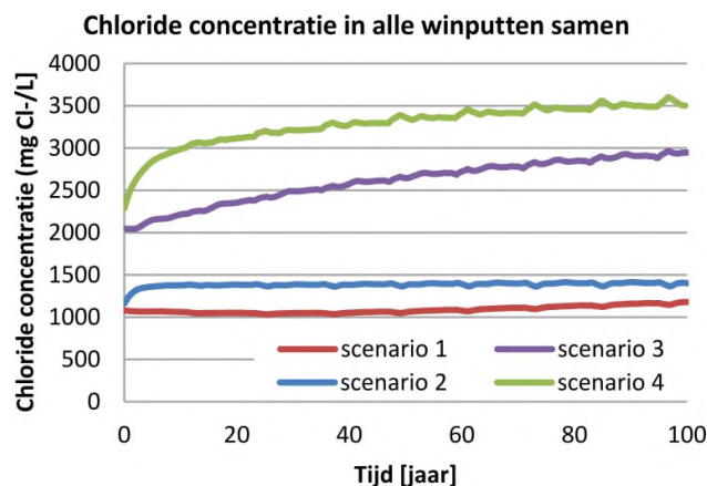
FIGUUR 4-27. ZOUTCONCENTRATIE OVER DE KOMENDE 100 JAAR IN ALLE WINPUTTEN VOOR SCENARIO 1, 2, 3 EN 4 OP DEZELFDE RUIMTELIJKE LOCATIES (MET ALS VERSCHIL DAT DE WINPUTTEN VAN SCENARIO 3 EN 4 DIEPER LIGGEN).
